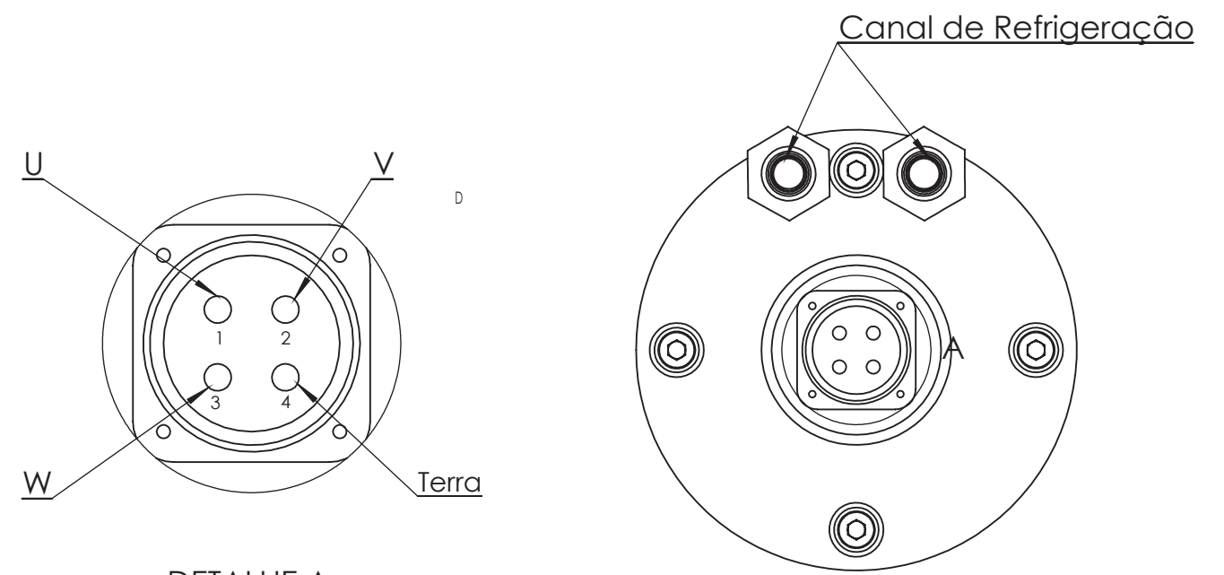
DETALHE A ESCALA 2 : 1
